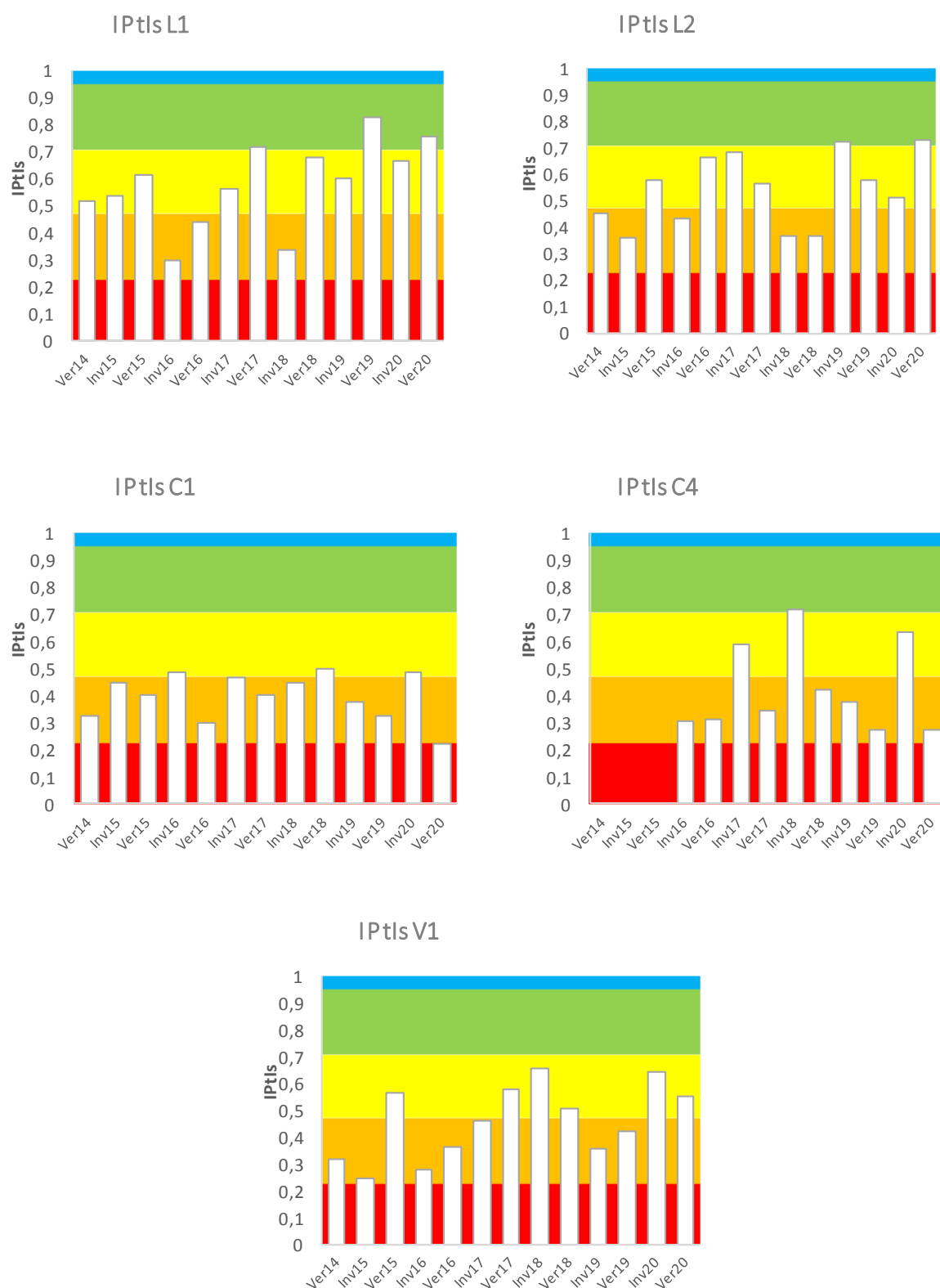
Figura 27 – Índice Português de Invertebrados do Sul, IPTIs (INAG, 2009) anual nas 5 unidades de amostragem. (Azul – excelente; Verde – Bom; Amarelo – Razoável; Laranja – Medíocre; Vermelho – Mau)
