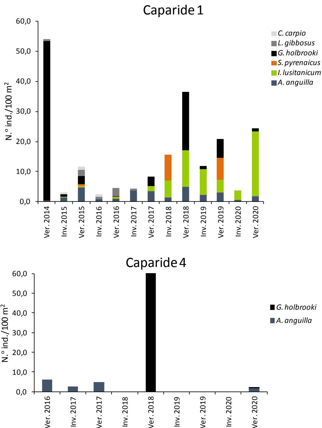
Figura 14 – Variação temporal da abundância relativa (N.º de Indivíduos capturados por 100 m²) por espécie em cada UA da ribeira de Caparide, entre junho de 2014 e junho de 2020. Gráficos relativos às UA 2 e 3 não representados por serem unidades descontinuadas (ver Ribeiro, 2017).
